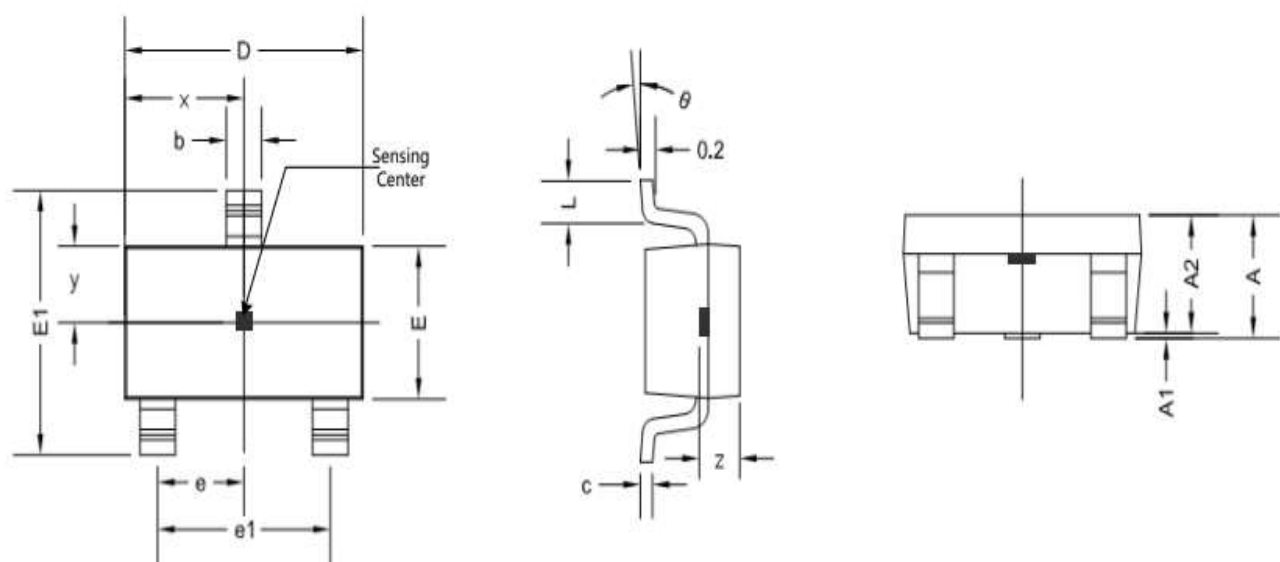
SOT23-3L 封装尺寸
